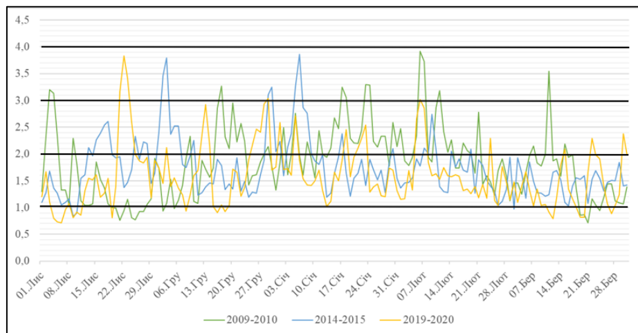
Рис. 6. Графік часового ходу показника S у листопаді-березні 2009-2010, 2014-2015 та 2019-2020 років
