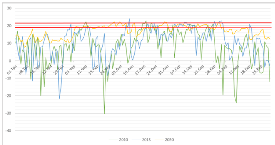
Рис. 1. Графік часового ходу показника ЕЕТ у травні-вересні 2010, 2015 та 2020 років
